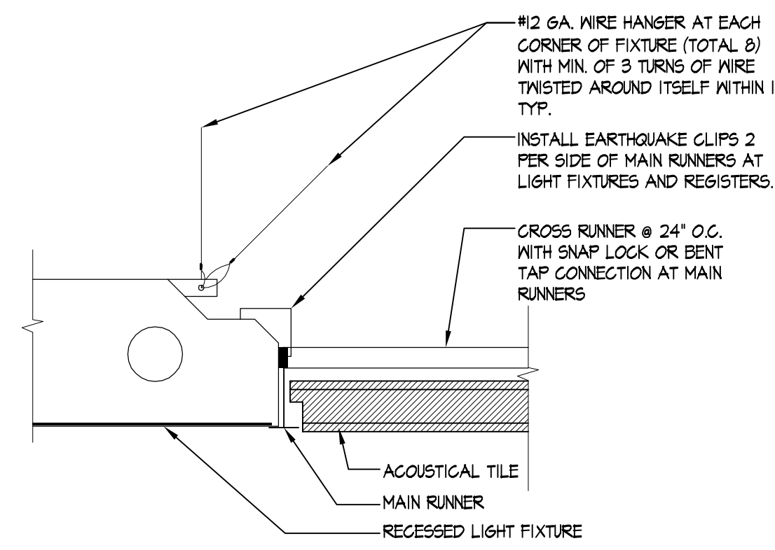
2 LIGHT FIXTURE DETAIL SCALE: N.T.S.
